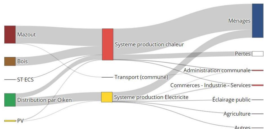
Diagramme des flux énergétiques de l'année 2020 sur le territoire communal de Grimisuat
